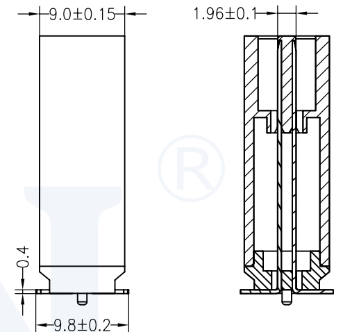
A-A SECTION
