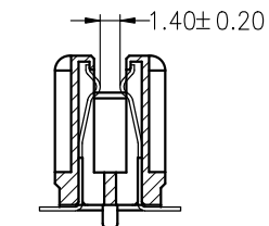
A-A SECTION
